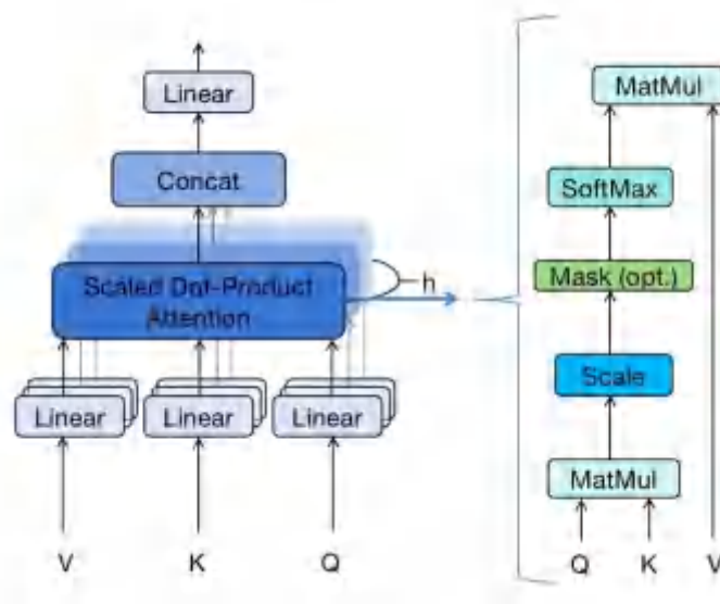
图 2-2 Transformer 自注意力网络[13]
