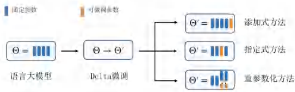
图 2-6 参数高效微调的 3 种范式[40]
