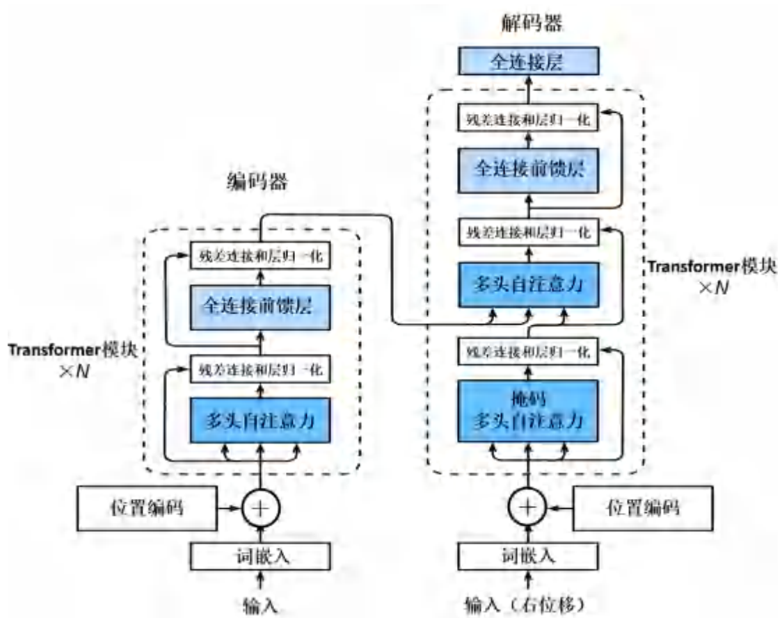
图 2-1 Transformer 架构[13]
