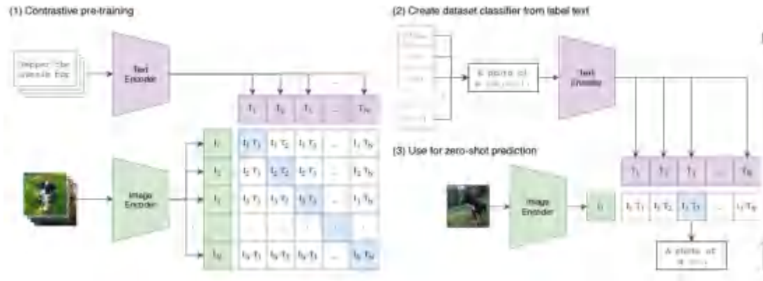
图 3-1 CLIP[65]模型架构图
