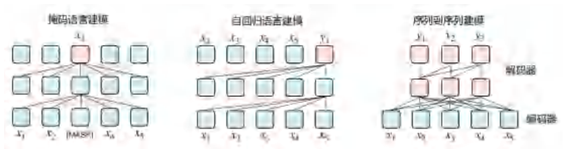
图 2-3 语言大模型的三种典型架构[36]
